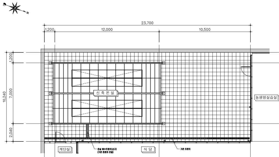
1 확대 배치도 축척: 1/100
